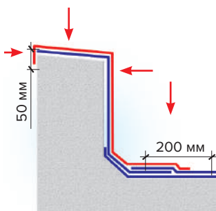
Рис.2. Кровля с наплавлением нижнего слоя
