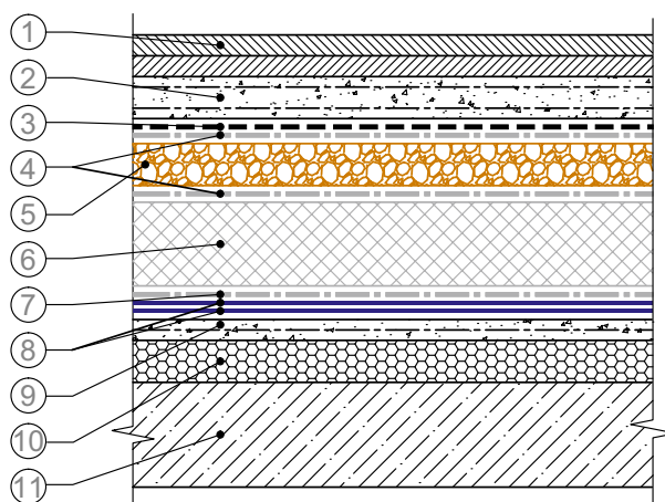
Рис. 6.2. Система ТН-КРОВЛЯ Авто:
