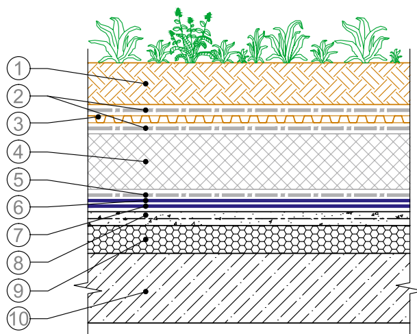
Рис. 6.3. Система ТН-КРОВЛЯ Грин:
