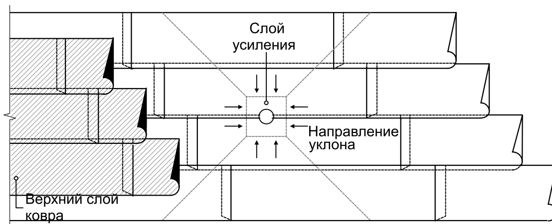
Рис. 10.2. Раскладка полотнищ кровельных материалов в районе водоприемной воронки
