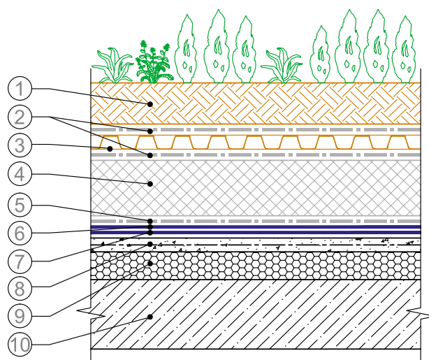
Рис. 6.4. Система ТН-КРОВЛЯ Грин Интенс:
