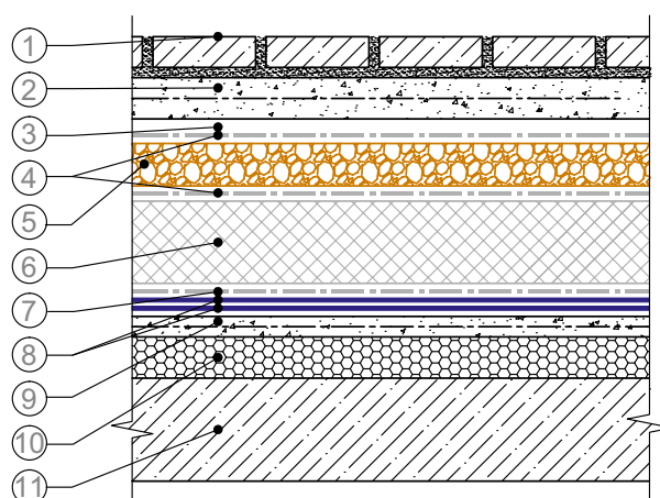
Рис. 6.1. Система ТН-КРОВЛЯ Тротуар:
