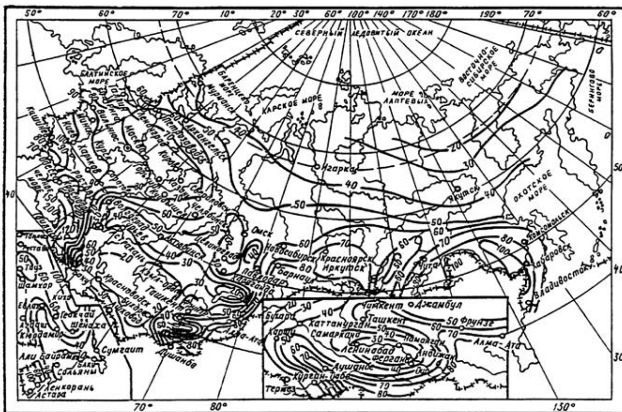
Рис. 1. Значения величин интенсивности дождя q_{20}
