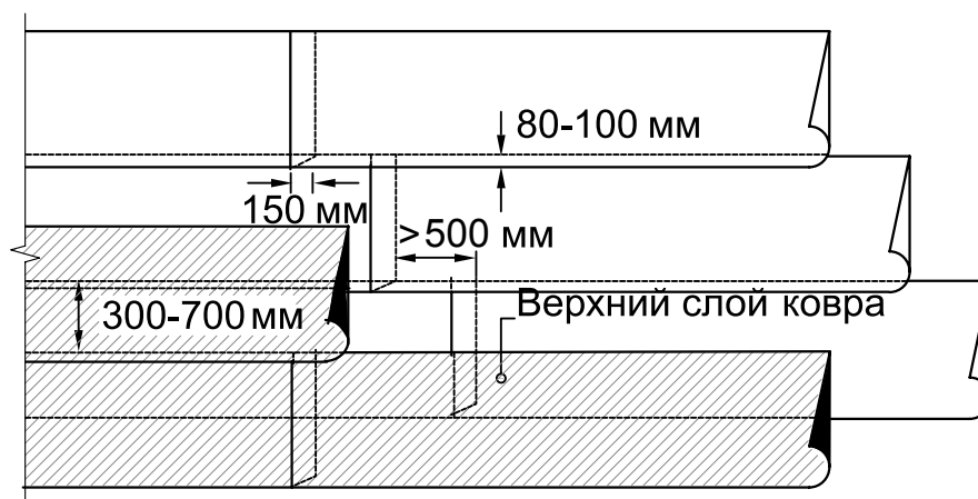
Рис. 10.4. Смещение полотнищ кровельного материала в смежных слоях
