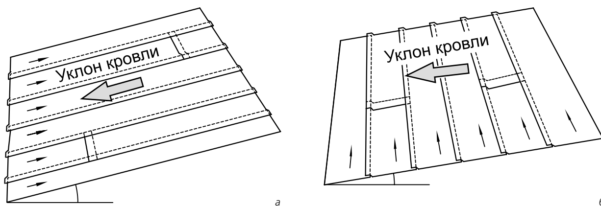
Рис. 10.1. Варианты укладки материала на скате крыши: а – направление укладки материала вдоль уклона; б – направление укладки материала перпендикулярно уклону
