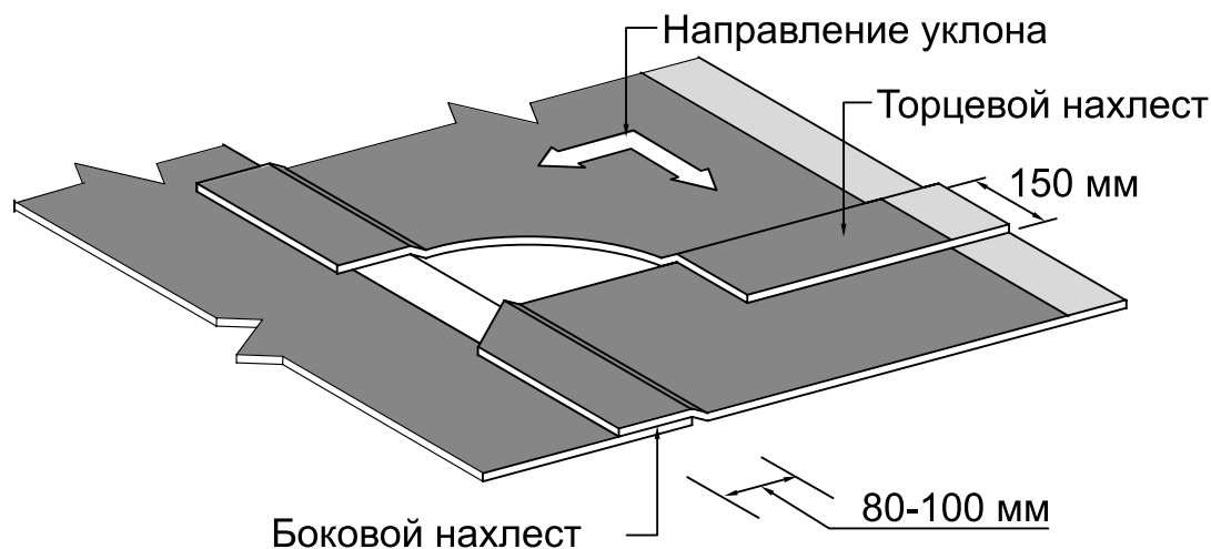
Рис. 10.3. Нахлесты полотнищ рулонного материала
