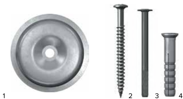
Рис. 7.41. Крепежные элементы при укладке водоизоляционного ковра по жесткому основанию:
