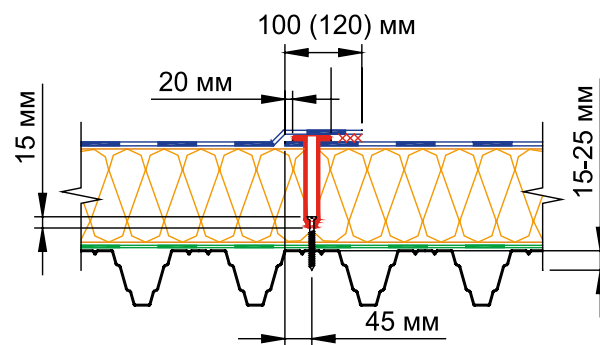
Рис. 7.42. Механическая фиксация материала в боковом нахлесте
