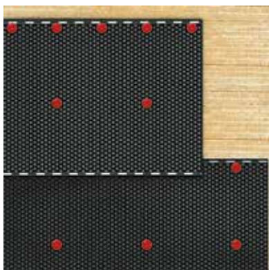
Рис. 7.43. Установка крепежа по центру материала Техноэласт ФИКС
