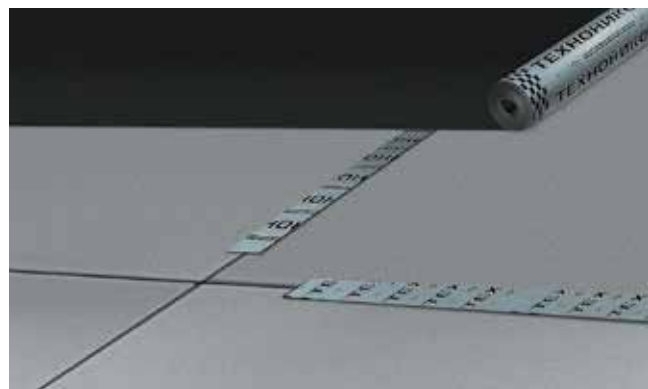
Рис. 7.16. Укладка полосок компенсаторов по температурно-усадочным швам
