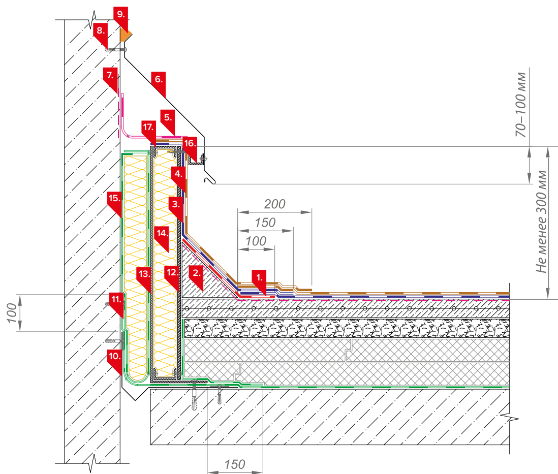
Рис. 7.55 . Тип Д. Деформационный шов в месте сопряжения двух разновысоких частей здания:
