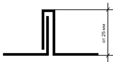
Рис. 7.27. Одинарный стоячий фальц
