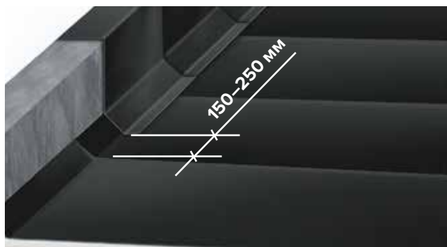
Рис. 7.19. Укладка нижнего дополнительного слоя на парапет
