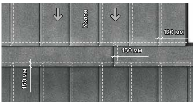
Рис. 7.48. Решение с выполнением сборной полосы
