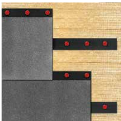
Рис. 7.44. Крепление полосы при устройстве однослойной кровли
