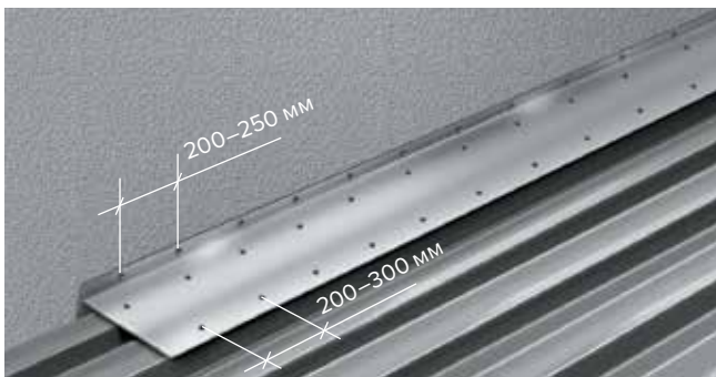
Рис. 7.3 Крепление L-образного элемента
