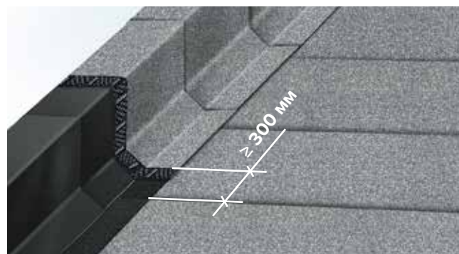
Рис. 7.20. Укладка верхнего дополнительного слоя на парапет
