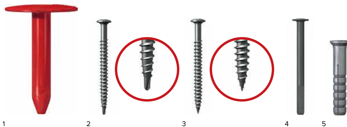
Рис. 7.40. Крепежные элементы при фиксации водоизоляционного ковра через теплоизоляционный слой
