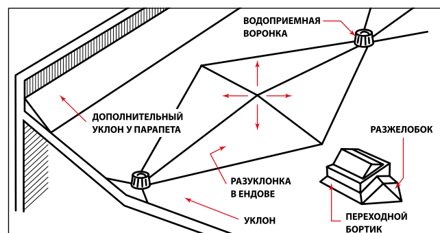
Рис. 7.11. Формирование уклона на крыше
