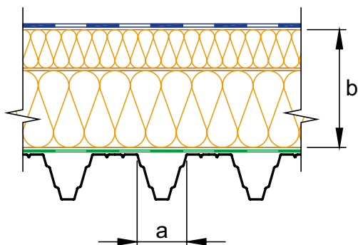
Рис. 7.9. Соотношение толщины утеплителя и расстояния между гофрами профлиста ( b \geq a/2 )
