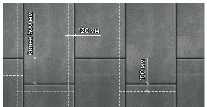
Рис. 7.49. Традиционное решение с разбежкой торцевых швов
