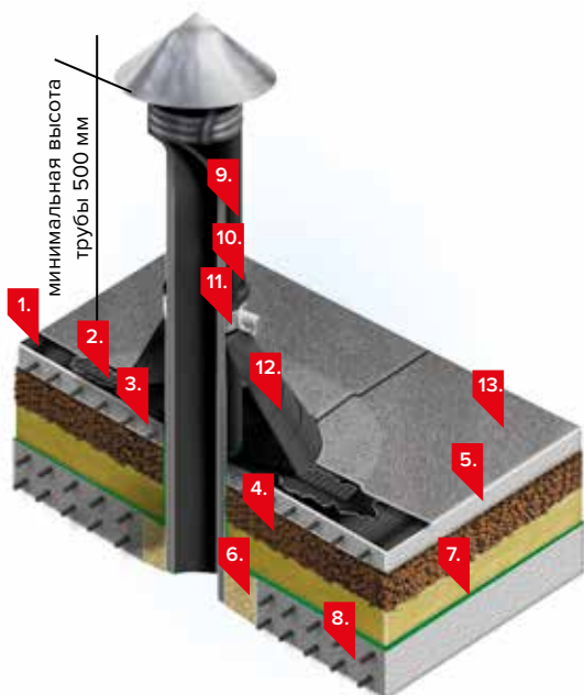
Рис. 7.31. Примыкание кровли к трубе с помощью эластичного переходника:
