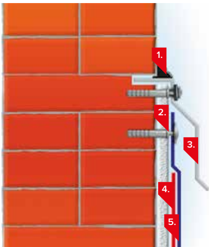
Рис. 7.25. Устройство узкой штробы
