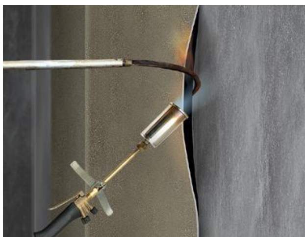
Рис. 4.10. Устройство слоя усиления внешнего угла
