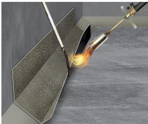
Рис. 4.7. Устройство слоя усиления при переходе с горизонтальной поверхности на вертикальную
