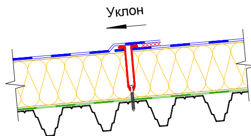
Рис. 5.18 «Встречный» шов
