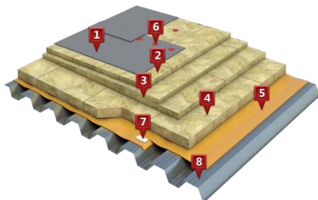
Рис. 4.1. Конструкция системы ТН-КРОВЛЯ Классик
