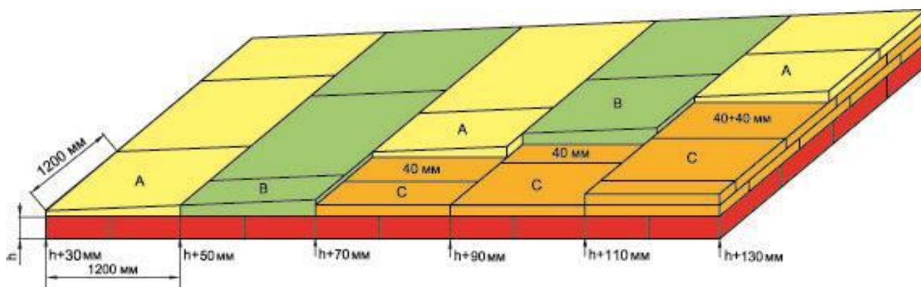
Рис. 5.5. Пример выполнения основного уклона из плит ТЕХНОРУФ Н30-КЛИН 1,7%
