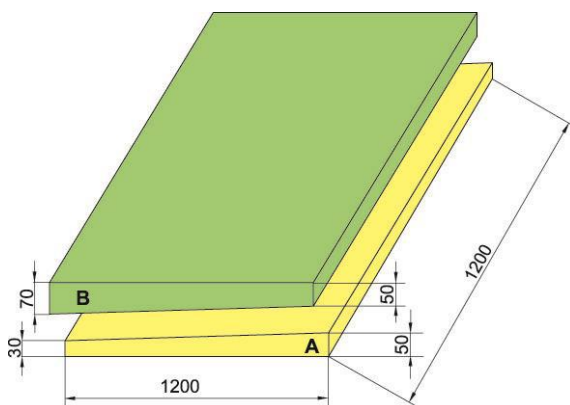
Рис. 5.4. Набор плит ТЕХНОРУФ Н30-КЛИН 1,7%
