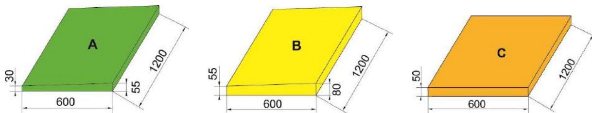
Рис. 5.6. Набор плит ТЕХНОРУФ Н30-КЛИН 4.2%
