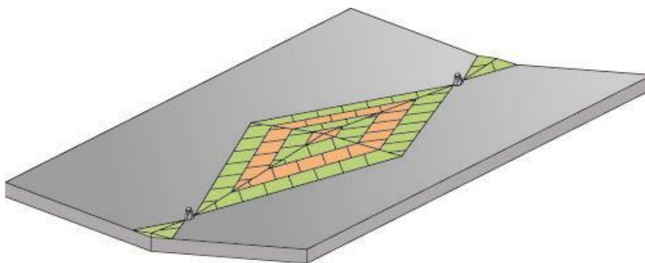
Рис. 5.7. Схема крепления теплоизоляционных плит
