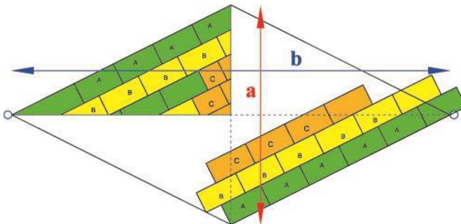
Рис. 5.8. Схема раскладки плит ТЕХНОРУФ Н30-КЛИН 4,2 % при создании разуклонки между воронками в ендове
