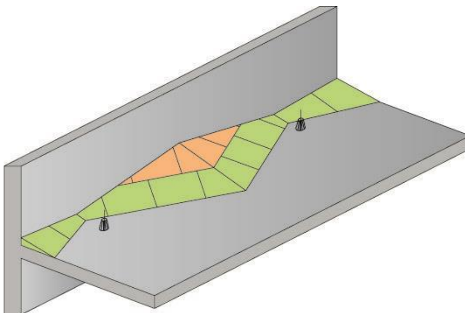
Рис. 5.9 Схема раскладки плит ТЕХНОРУФ Н30-КЛИН 4,2 % при устройстве контруклона в парапетной зоне
