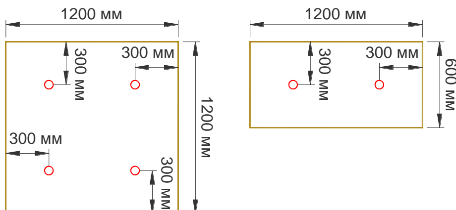
Рис. 5.11. Схема крепления теплоизоляционных плит из минеральной ваты
